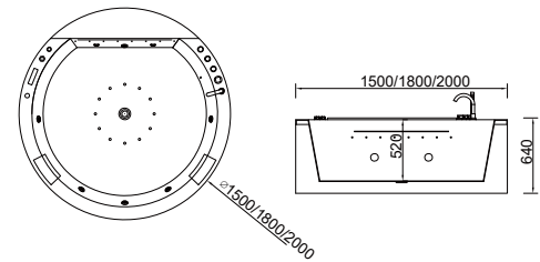
Q430B 1500*1500*640mm , 1800*1800*640mm 2000*2000*640mm
