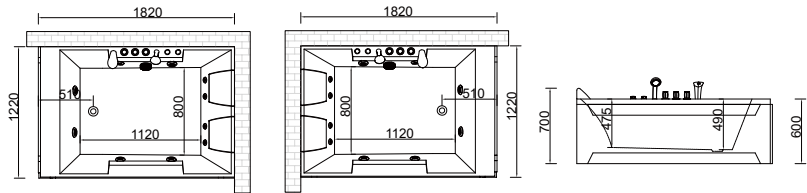
Q367(L/R) 1820*1220*600mm
