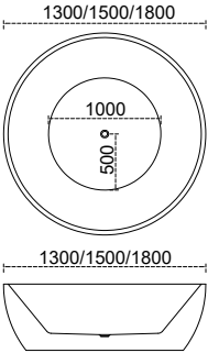
Q196 1300×1300×600mm, 1500×1500×600mm, 1800×1800×600mm
